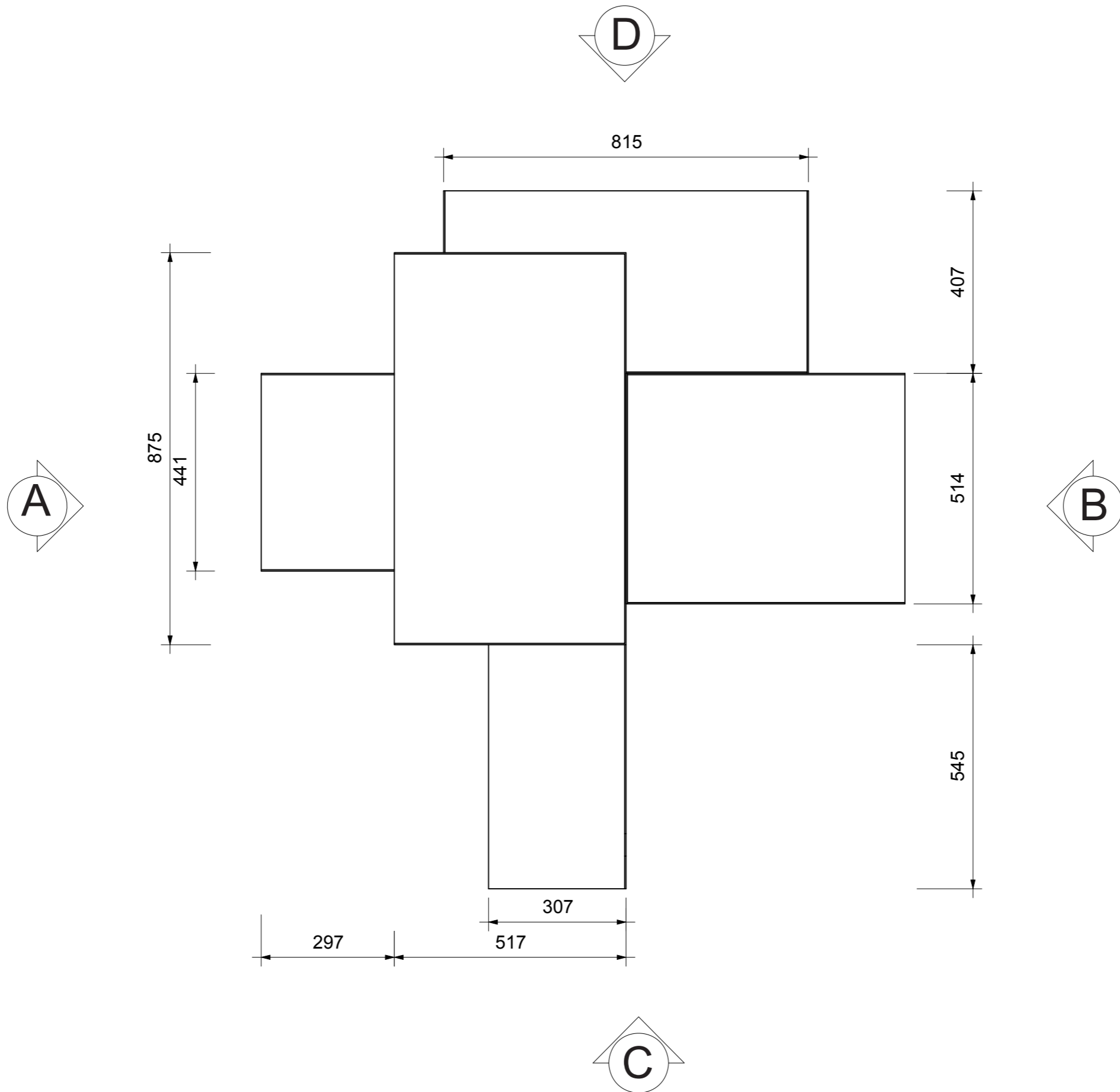
PIANTA 1:10
