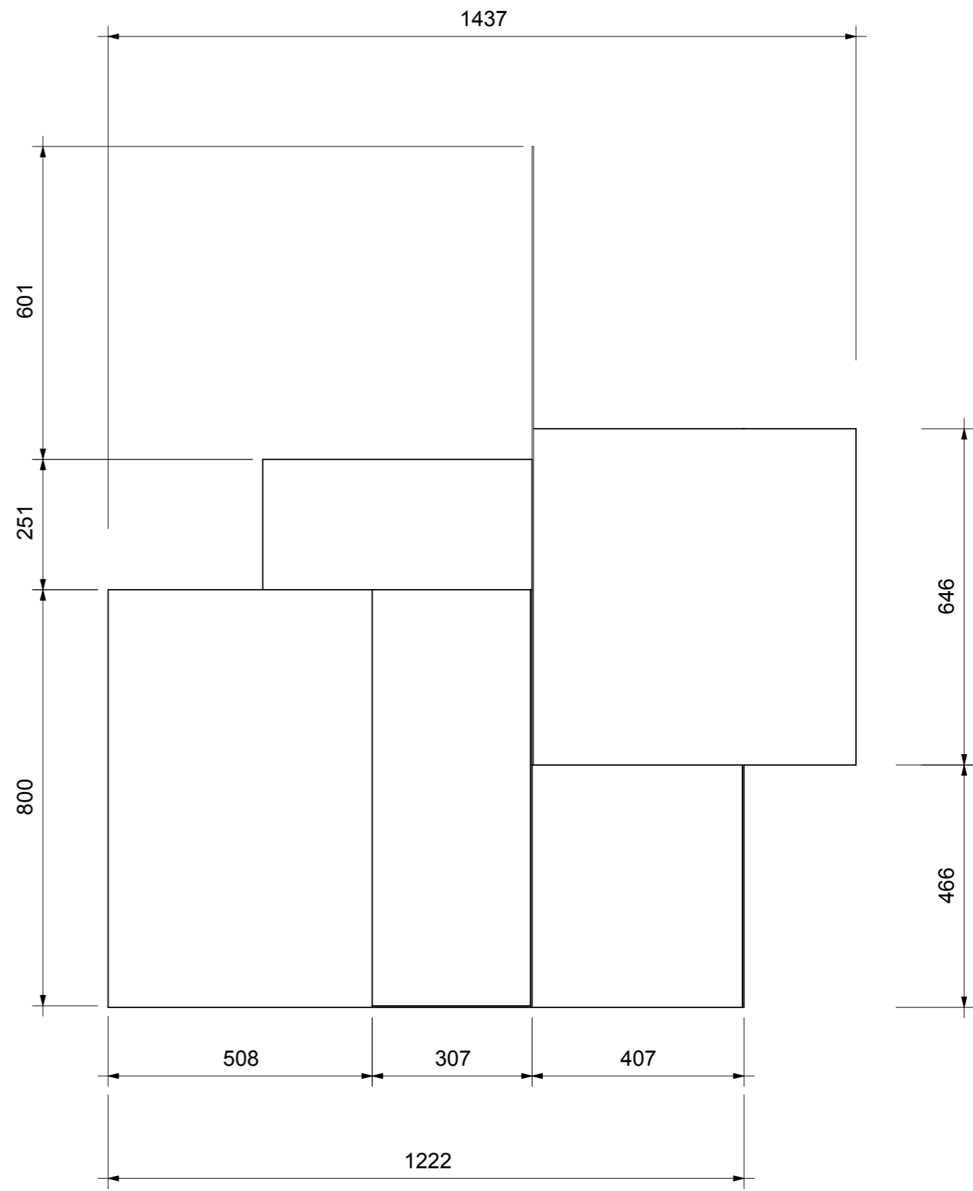
PROSPETTO D 1:10
