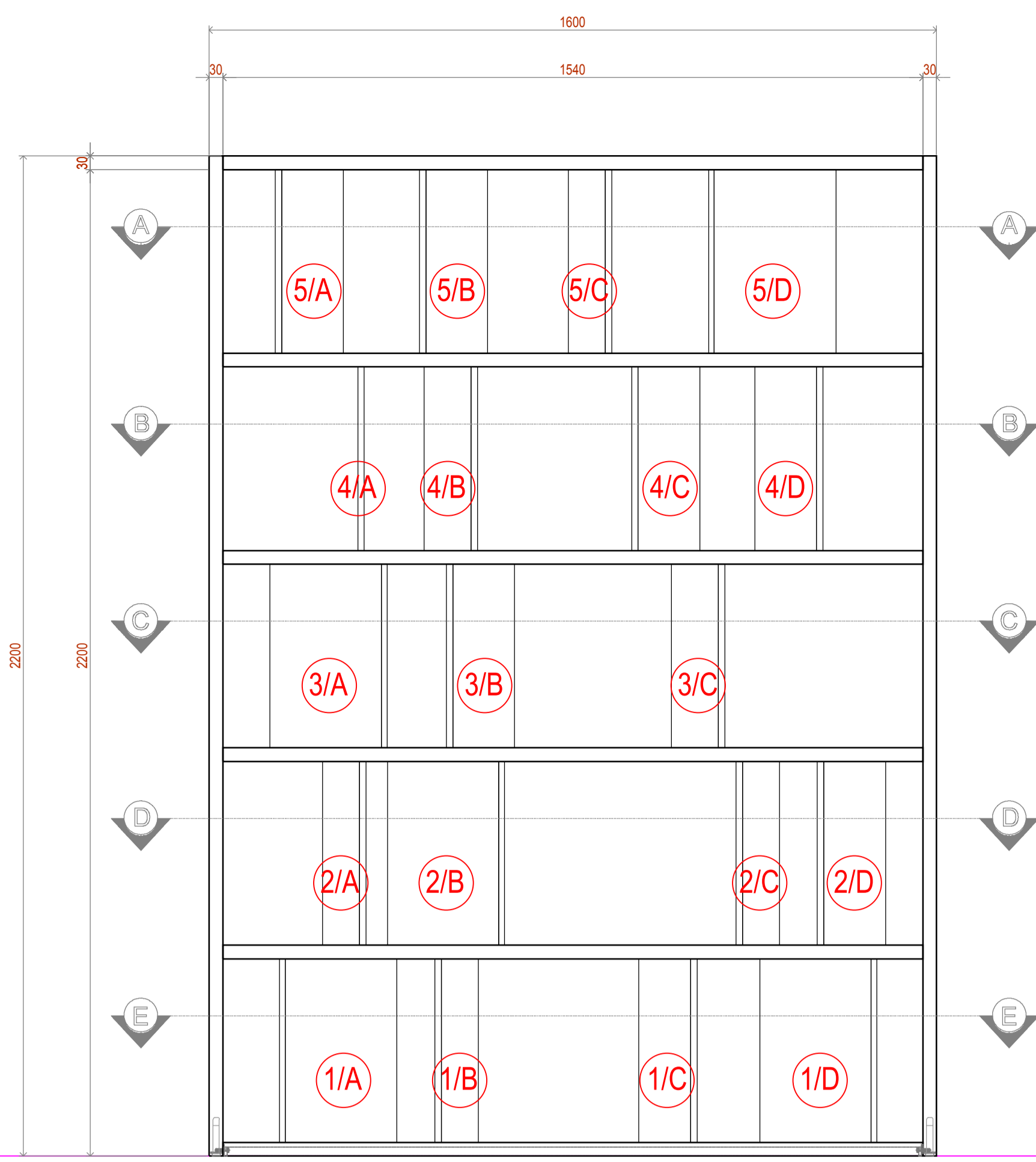
FRONTE - 1:10
