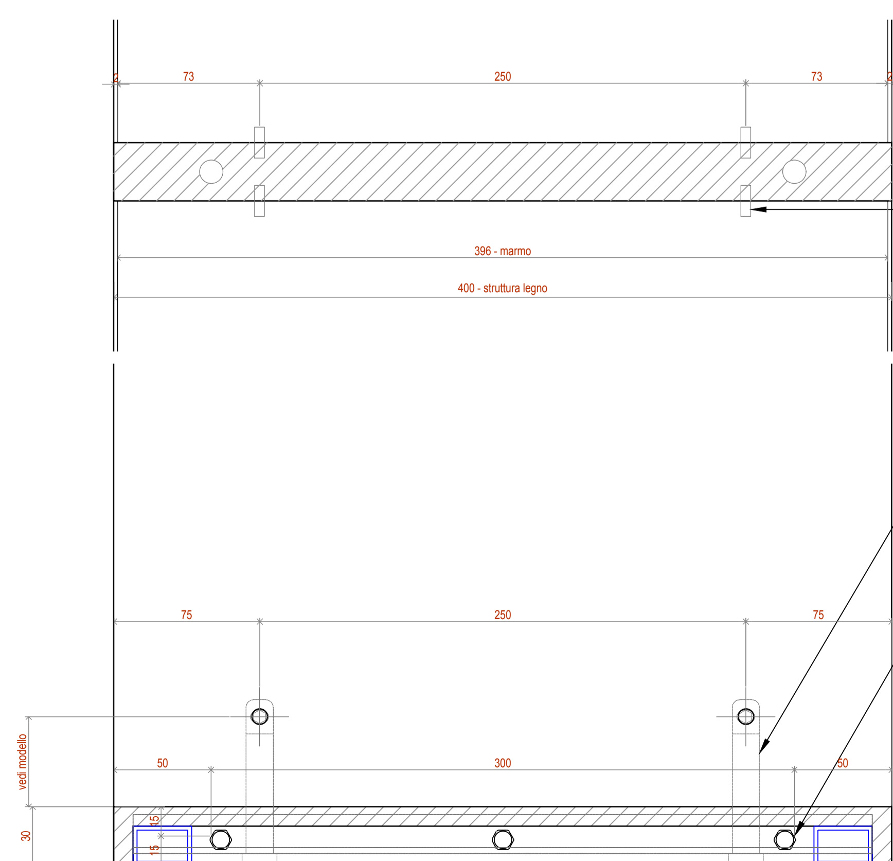
DETTAGLIO FORATURE - 1:2
