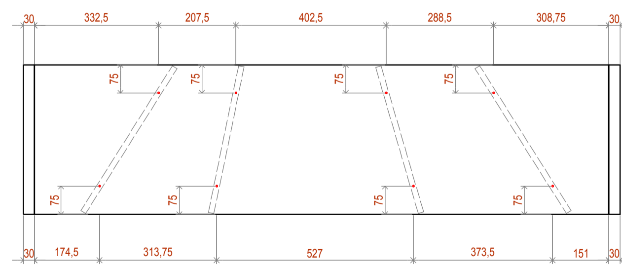
SCHEMA FORATURE SPINE NYLON PER DIVISORI IN MARMO - 1:10
