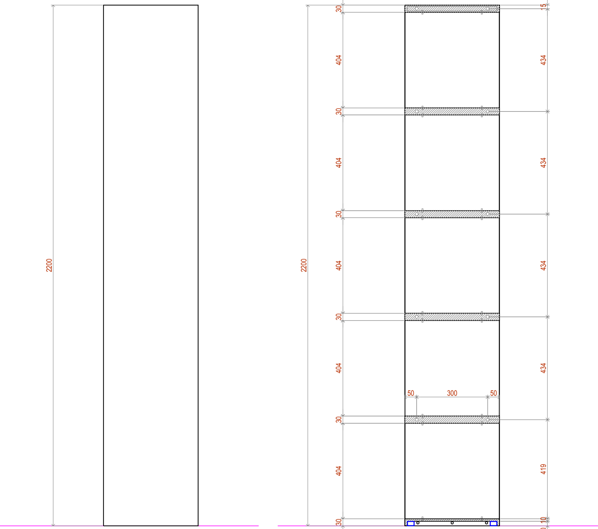
FIANCO - 1:10
